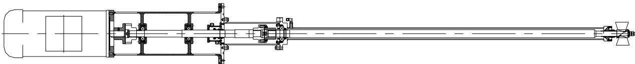
Particolari interno e lanterna agitatore per mescolatore da L 3500 Interior details and mixer's lantern for 3,500 L mixer
